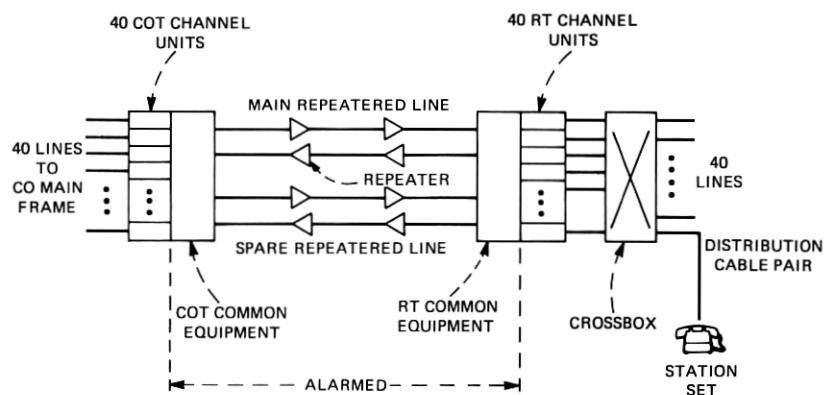
Fig. 1— SLC ™-40 system block diagram.
